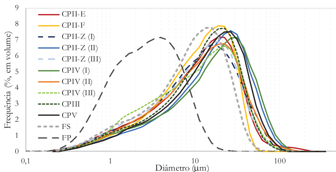
Figura 1 Curvas granulométricas dos cimentos e fillers utilizados
